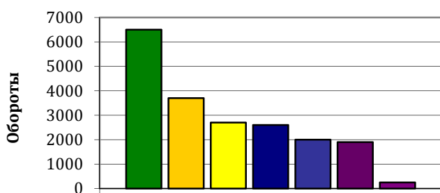
Показатели износостойкости различных типов лаков по тесту Табер EN13329
